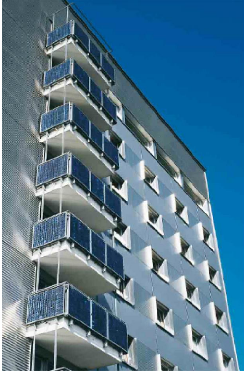
شكل (4-18) خلايا شمسية كدريزين البلكنات والتراسات (Krawietz, 2011)
