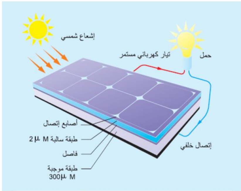
شكل (2-3) انتاج الخلايا الشمسية للطاقة الكهربائية (محيسن، 2006)
